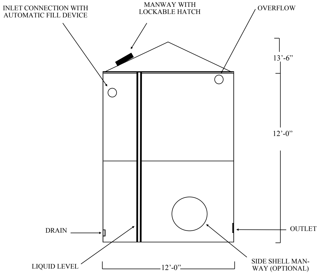
ELEVATION
